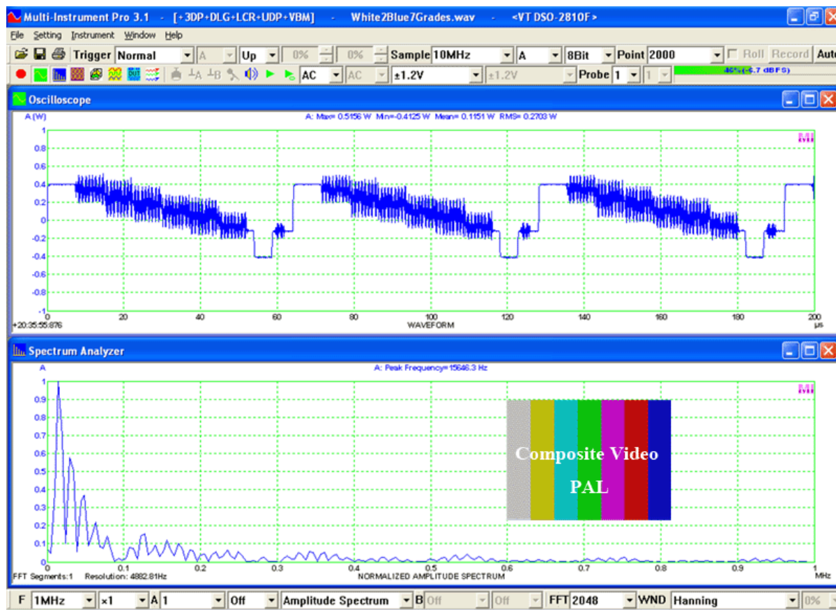
下图是测量一个 500Hz 的正弦波和一个 1kHz 的方波的结果。
